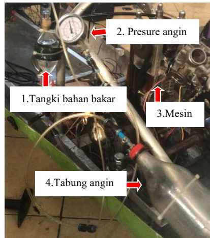
Gambar 2. Komponen mesin
