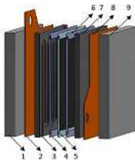
Gambar 2. Konfigurasi dari Satu Stack PEMFC
