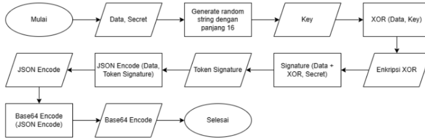
Gambar 2. Diagram Alir Proses Pembuatan Token
