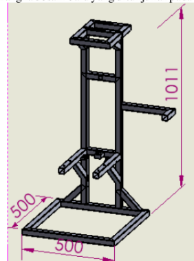
Gambar 3. Kerangka Mesin Desain Baru
