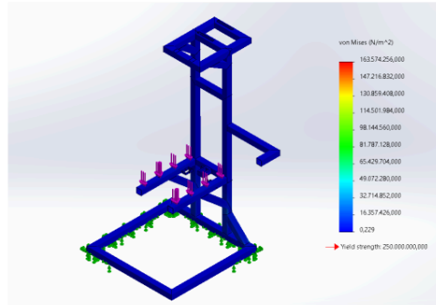
Gambar 6. Hasil Analisis Von Misses
