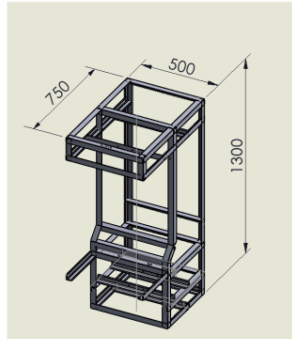
Gambar 2. Konsep Referensi Mesin Pencetak Bakso
