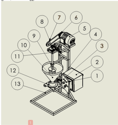
Gambar 5. Konsep Desain (B)
