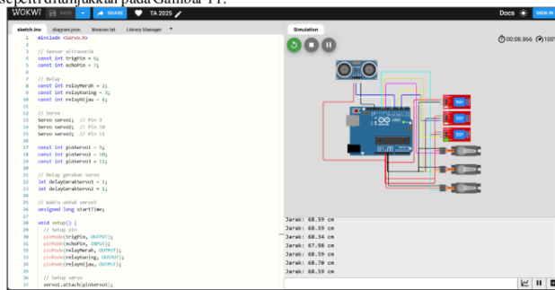
Gambar 11. Simulasi Dengan Wokwi
