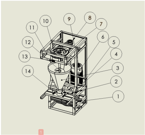
Gambar 4 . Konsep Desain (A)
