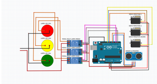
Gambar 10, Rangkaian Sistem Arduino Uno
