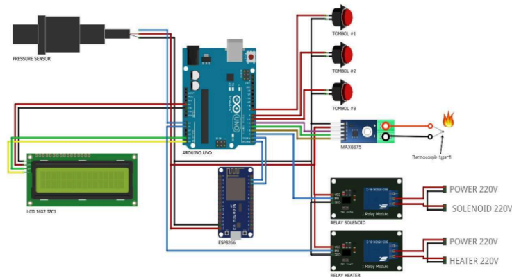
Gambar 3. diagram elektrik
