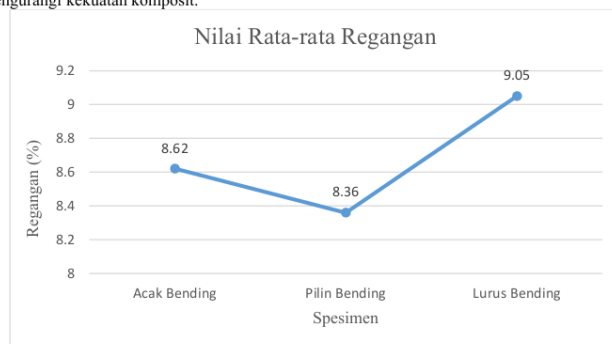
Gambar 16. Grafik Nilai Rata-Rata Regangan Uji Bending
