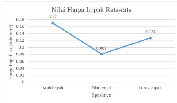
Gambar 12. Grafik Nilai Harga Impak Rata-Rata Uji Impak
