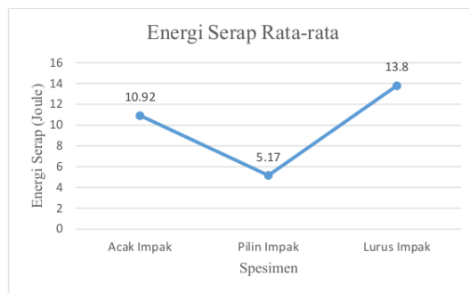
Gambar 11. Grafik Energi Serap Rata-Rata Uji Impact
