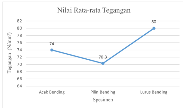
Gambar 15. Grafik Nilai Rata-Rata Tegangan Uji Bending
