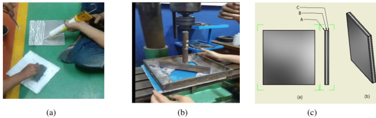
Gambar 2.6 (a) Pelengketan ACP (b) Pengepressan ACP (c) Skema Material ACP yang telah jadi
