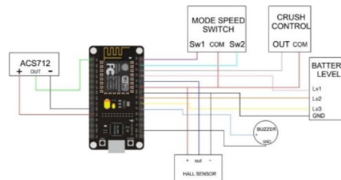
Gambar 5 design wiring alat keseluruhan
