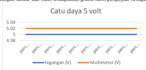
Gambar 8 Grafik Pengujian Catu daya 5 Volt
