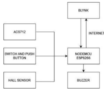
Gambar 1 arsitektur sistem
