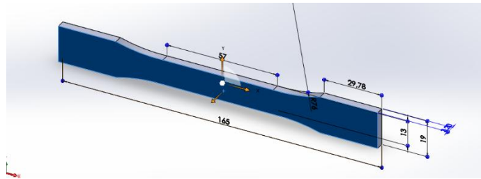
Gambar 3 Gambar 3D spesimen uji tarik
