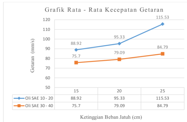
Gambar 4. Grafik Rata-Rata Kecepatan Getaran
