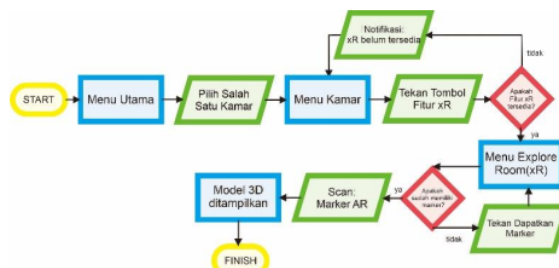
Gambar 3. Flowchart Aplikasi
