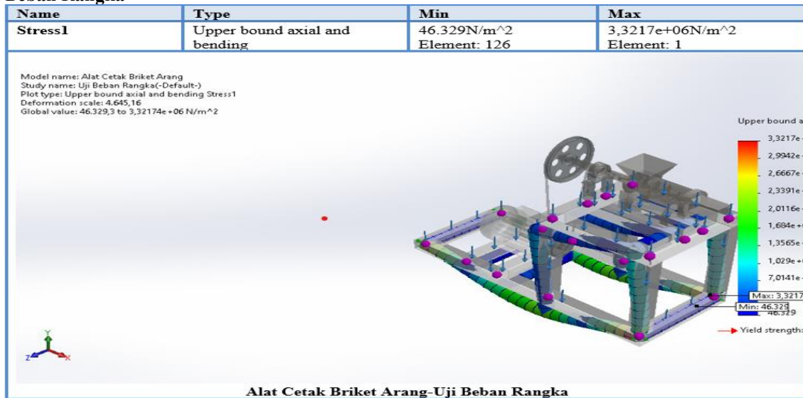
Gambar 12. Uji Beban Rangka
