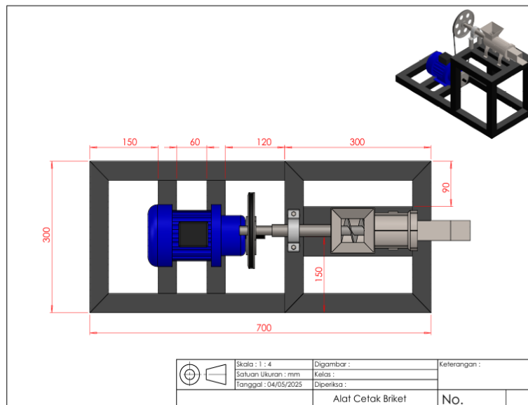
Gambar 4. Desain Atas Samping Mesin Arang Briket
