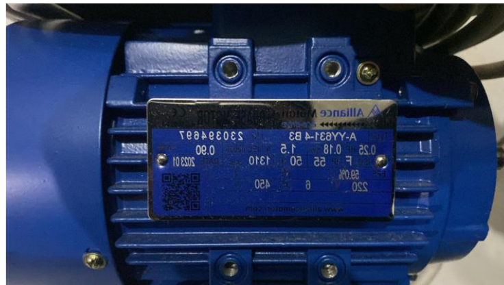
Gambar 10. Speksifikasi Motor
