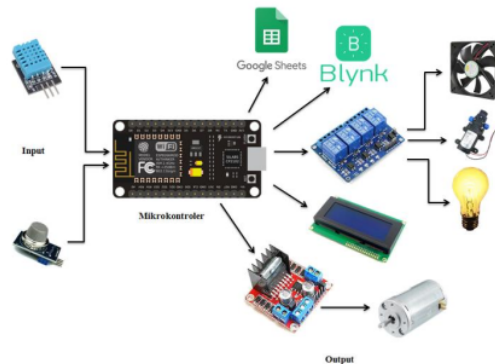
Gambar 1. Arsitektur Umum Sistem
