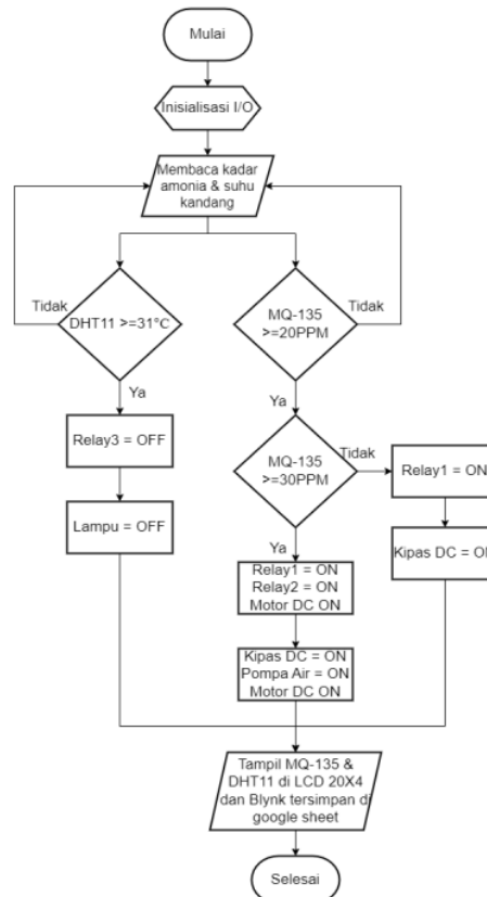
Gambar 5. Perancangan Sistem
