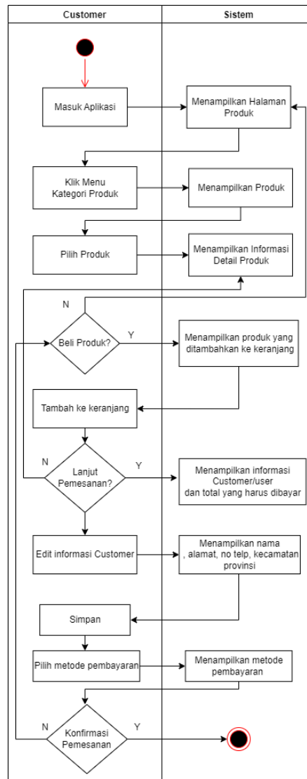
Gambar 7. Activity Diagram Order dan Pembayaran
