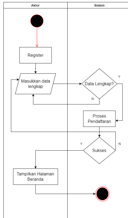
Gambar 4. Activity Diagram Melakukan Registrasi
