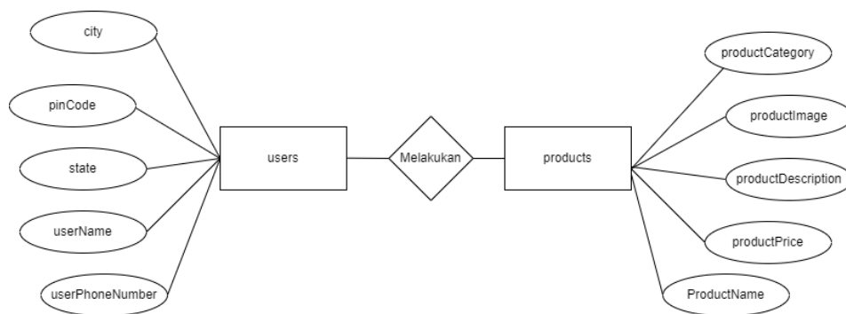
Gambar 9 . ER Diagram
