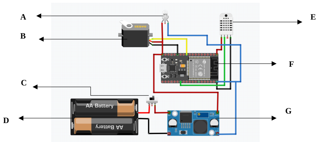
Gambar 3. Skema Rangkaian Monitoring suhu dan kelembaban
