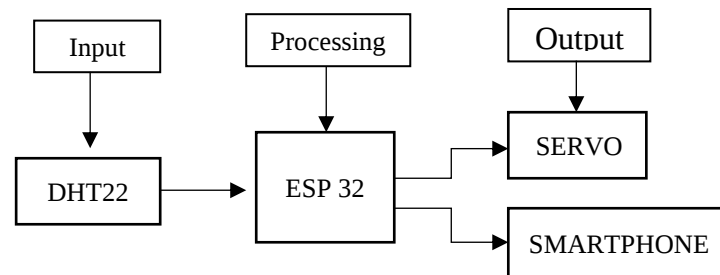
Gambar 1. Diagram Block Rangkaian Alat
