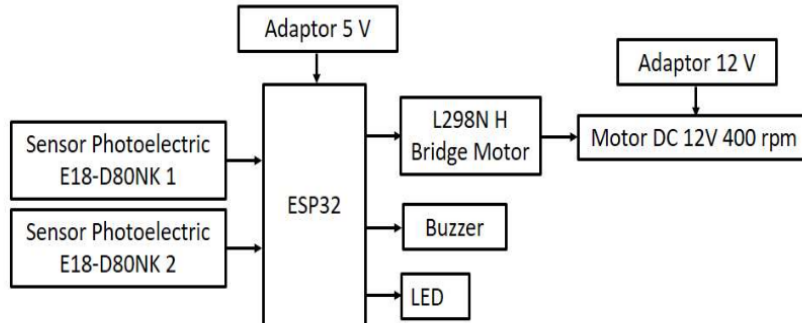
Gambar 1. Blok Diagram Sistem
