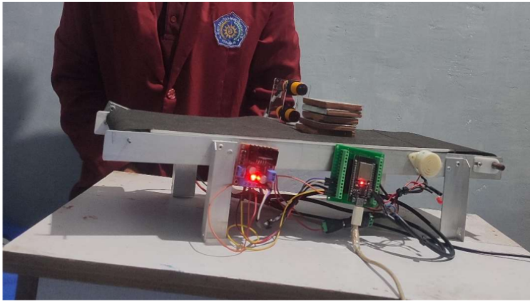
Gambar 8. Pengujian Rangkaian Keseluruhan Alat
