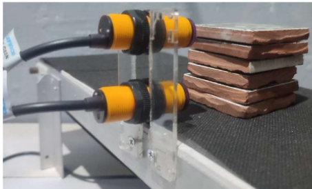
Gambar 5. Pengujian Sensitifitas Sensor Photoelectric E18-D80NK
