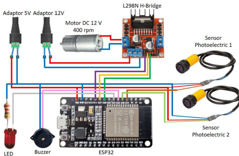
Gambar 4. Skema Rangkaian
