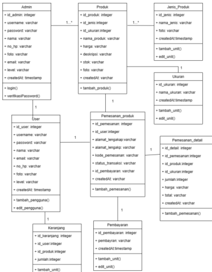
Gambar 4 Class Diagram Aplikasi Untuk Admin dan User
