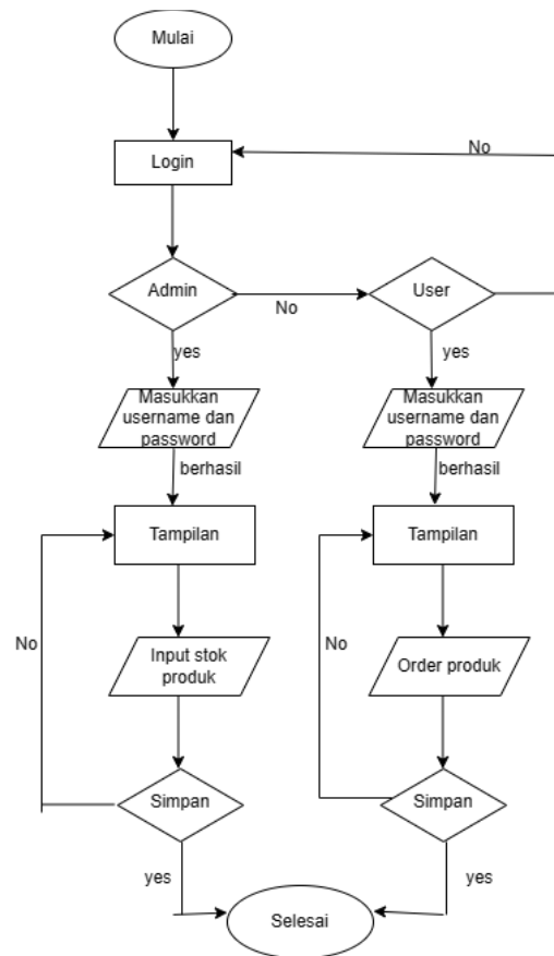
Gambar 2 Flowchart Aplikasi Untuk Admin dan User
