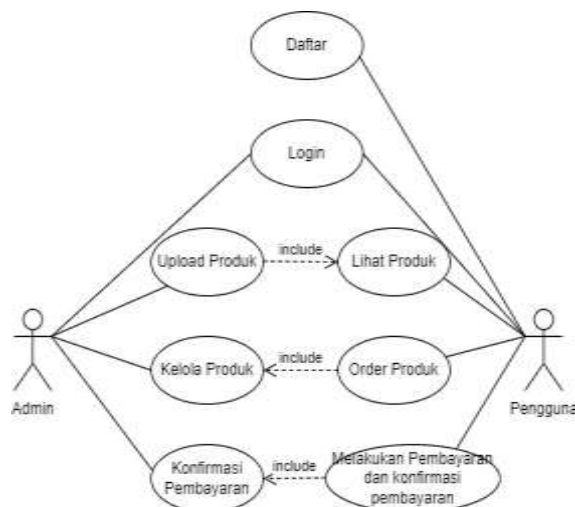
Gambar 3 Use Case Diagram Aplikasi Untuk Admin dan User
