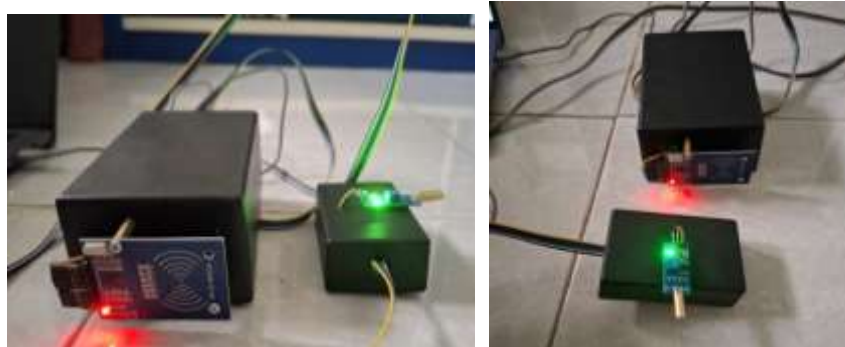
Gambar 5. Rangkaian ESP8266 dengan Sensor Tilt dan Sensor Accelero MPU6050
