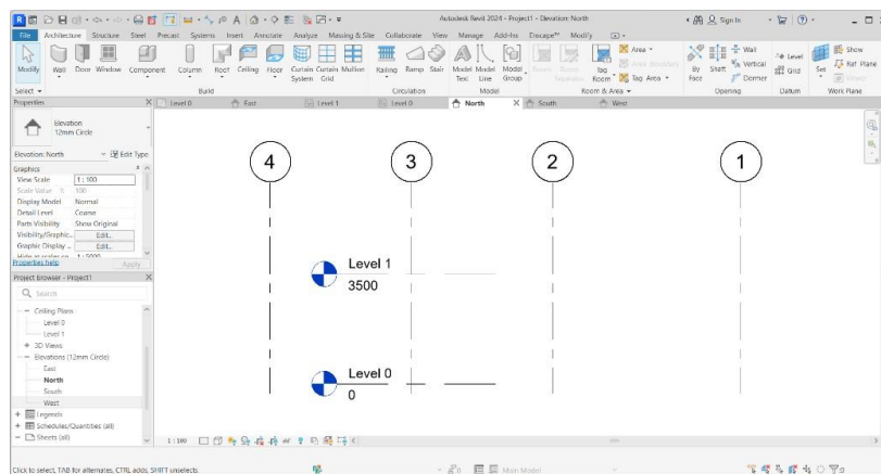
Gambar 5. Pembuatan Level [5]
