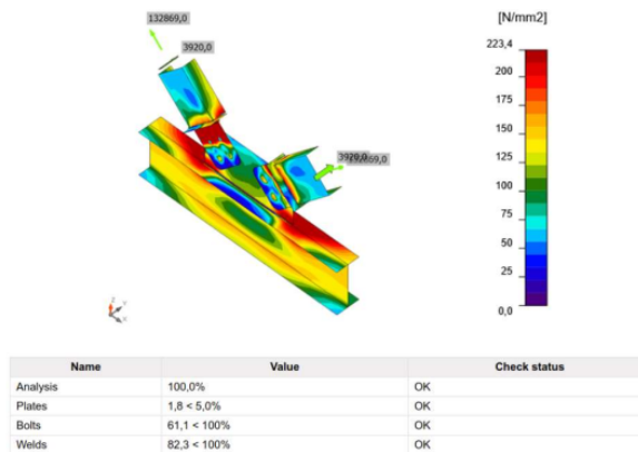
Gambar 10. Analisis sambungan 3
