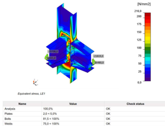
Gambar 6. Analisis sambungan 1
