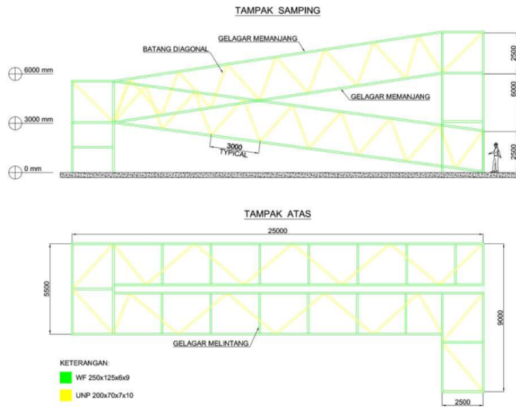
Gambar 1. Layout gangway
