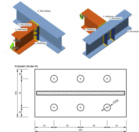
Gambar 7. Desain sambungan 2
