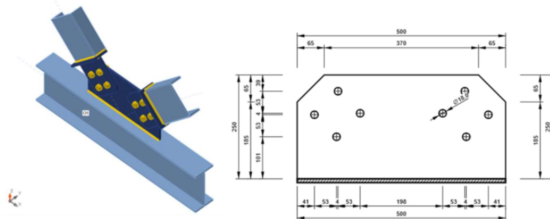
Gambar 9. Desain sambungan 3
