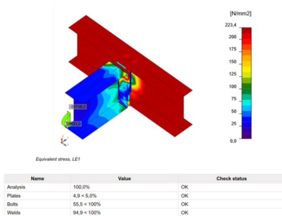
Gambar 8. Analisis sambungan 2
