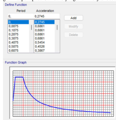
Gambar 3. Grafik respons spektra
