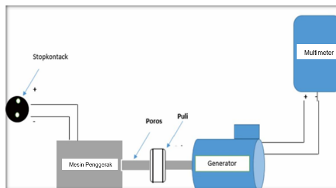
Gambar 5. Instalasi Pengujian Tanpa beban
