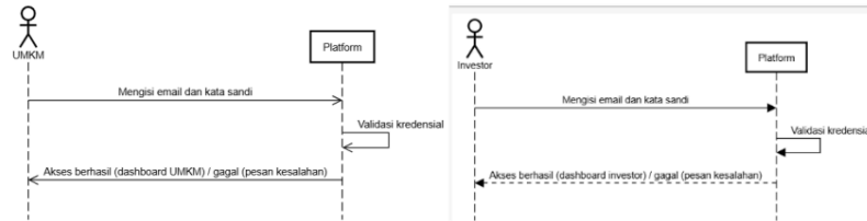
Gambar 3. Login
