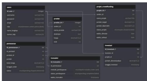
Gambar 11. Rancangan database
