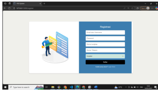
Gambar 18. Halaman Registrasi
