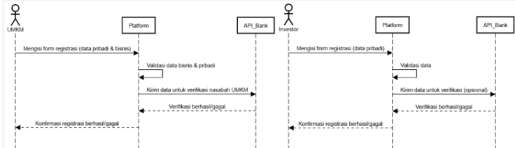
Gambar 2. Registrasi
