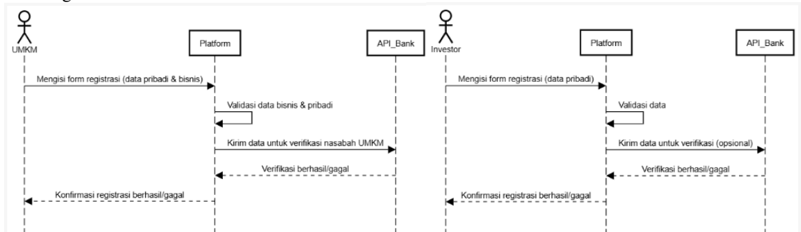
Gambar 2. Registrasi
