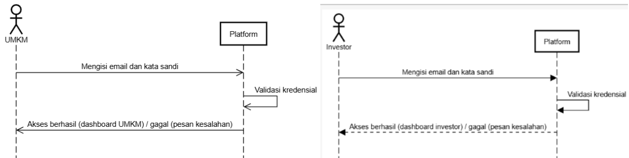
Gambar 3. Login
