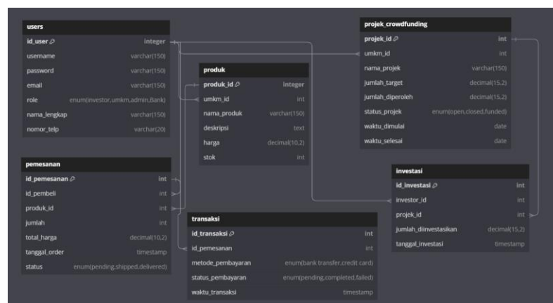
Gambar 11. Rancangan database
