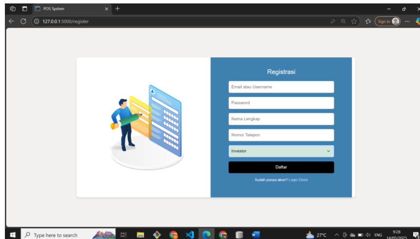
Gambar 18. Halaman Registrasi
