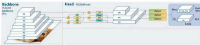
Gambar 5. Arsitektur YOLOv8
