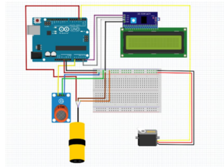
Gambar 4. Rangkaian Sistem Elektrikal
