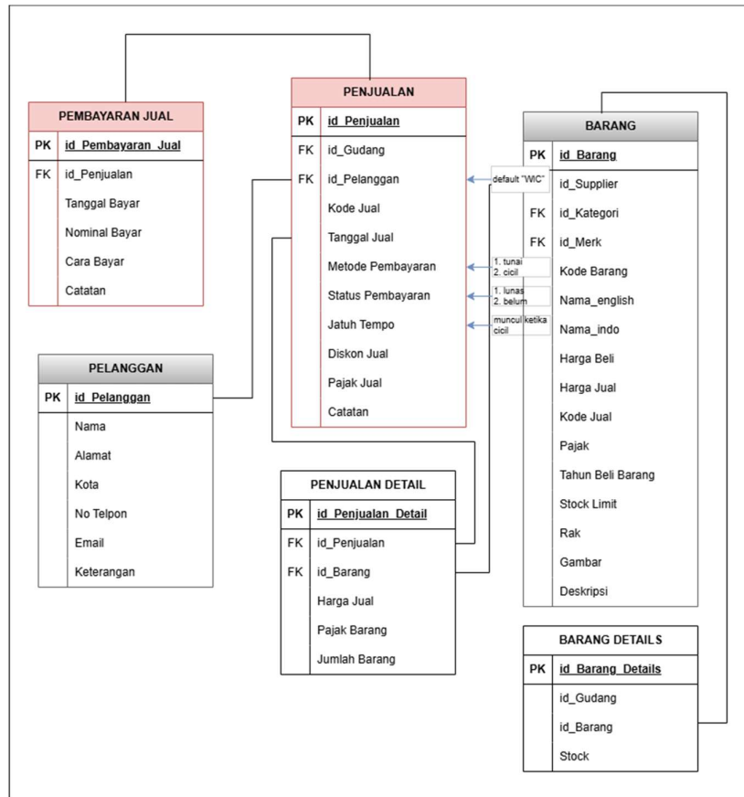
Gambar 5. PDM Penjualan
