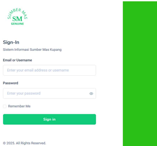
Gambar 14. Tampilan Login
