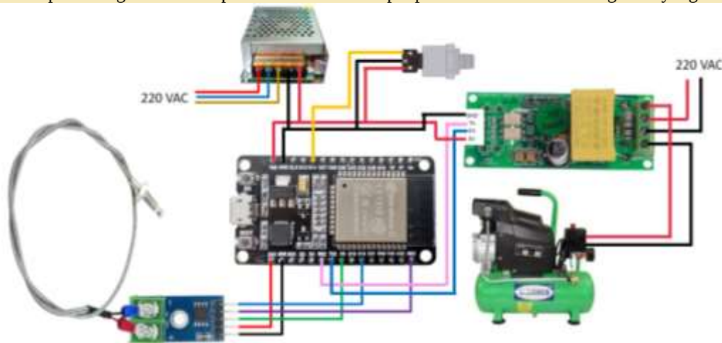
Gambar 5. Skema Rangkaian
