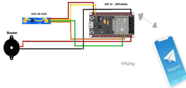
Gambar 3. rangkaian pendeteksi keberadaan manusia
