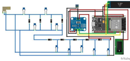
Gambar 2. Rangkaian sistem
