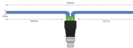
Gambar 2. Desain antena dipole
