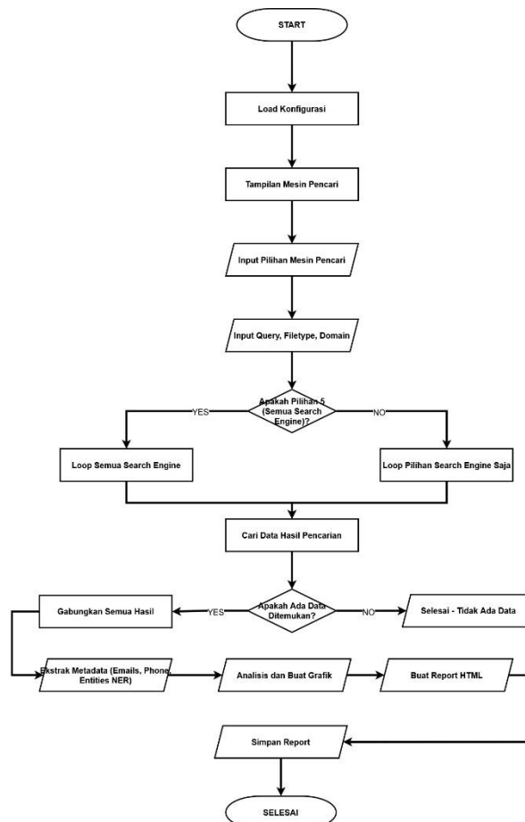
Gambar 2.1 Flowchart Arsitektur Tool OSINT.
