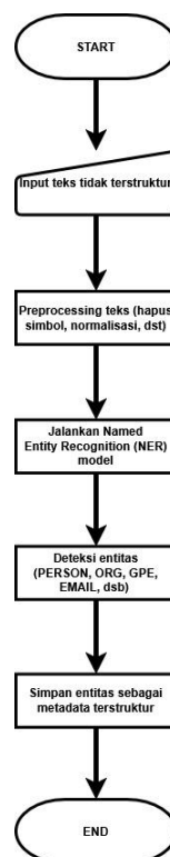
Gambar 2.2 Diagram ekstraksi metadata menggunakan Named Entity Recognition (NER).
