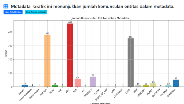
Gambar 3.4 Visualisasi jumlah kemunculan entitas dalam metadata.
