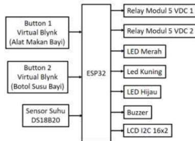
Gambar 1. Blok Diagram Sistem
