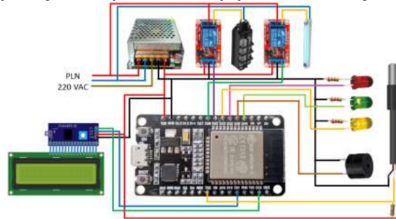
Gambar 5. Skema Rangkaian
