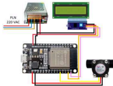
Gambar 6. Skema Rangkaian
