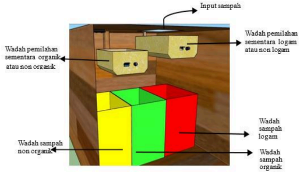
Gambar 4. Desain Alat
