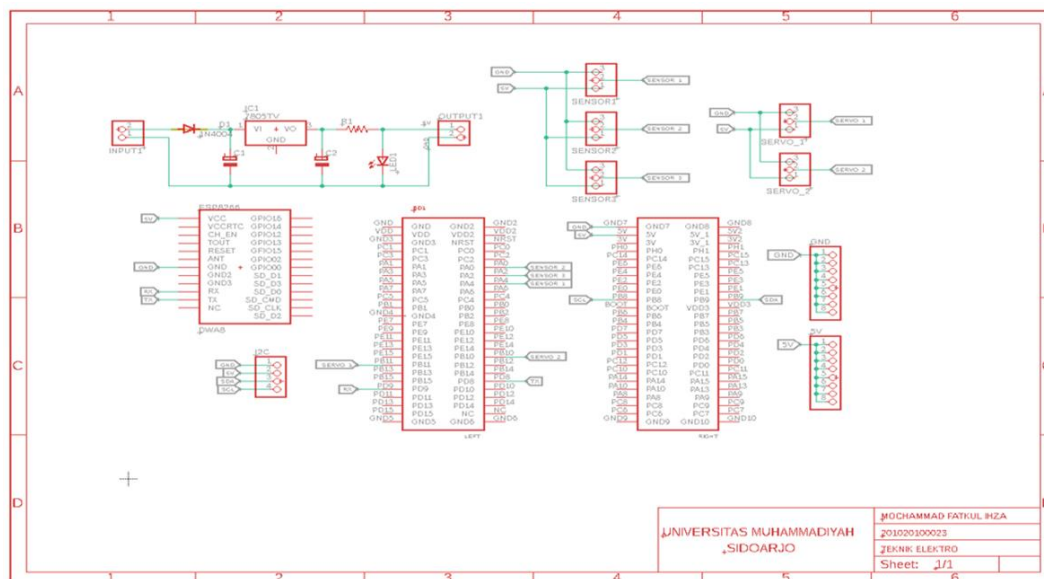
Gambar 3. Skema Rangkaian
