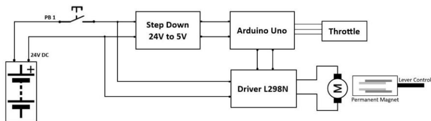
Gambar 3 Rangkaian kontrol
