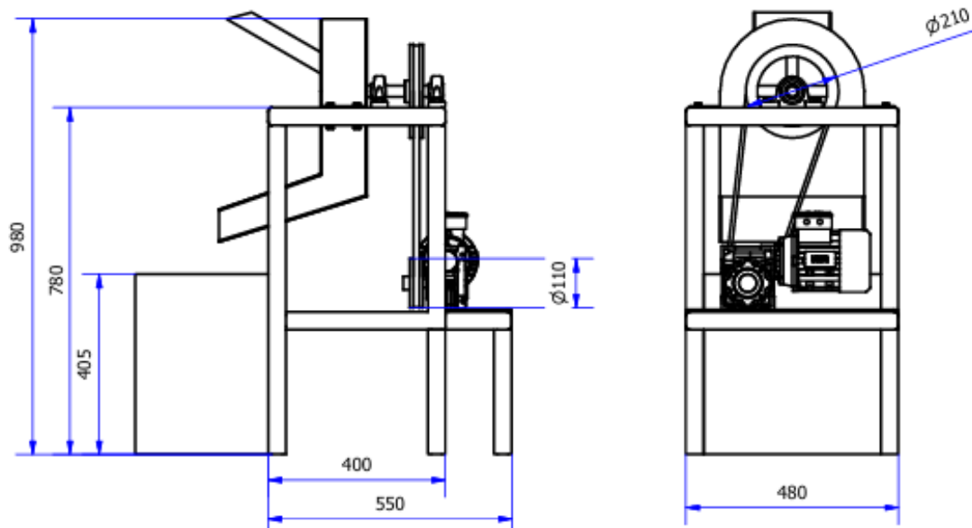
Gambar 2. Rancangan Alat Penyerut
