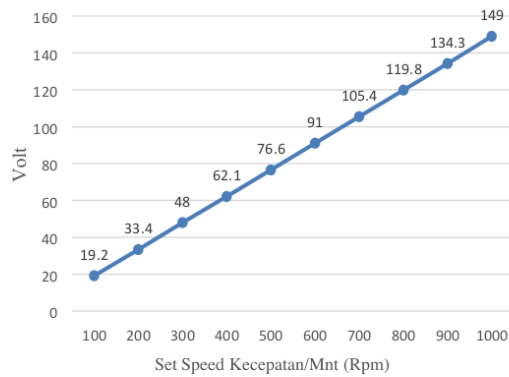
Gambar 7. Grafik Pengukuran Output Voltage
