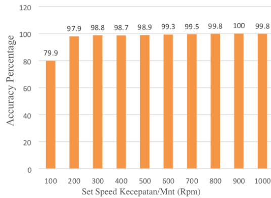
Gambar 8. Grafik Akurasi Output Voltage
