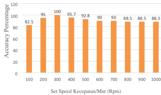
Gambar 10. Grafik Akurasi Output Current
