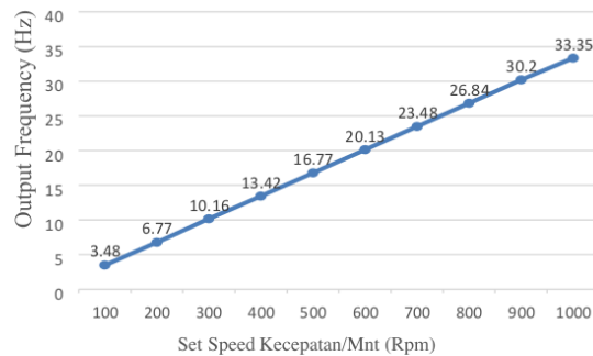
Gambar 5. Grafik pengukuran Frequency Terhadap Rpm Motor
