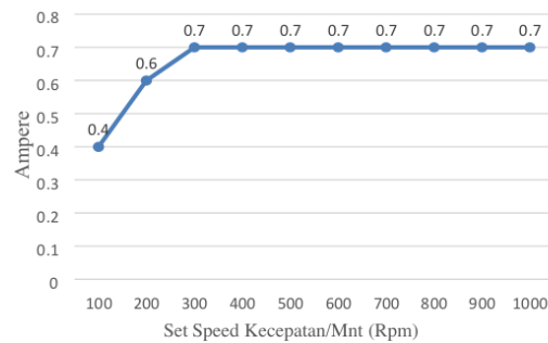
Gambar 9. Grafik Pengukuran Output Current
