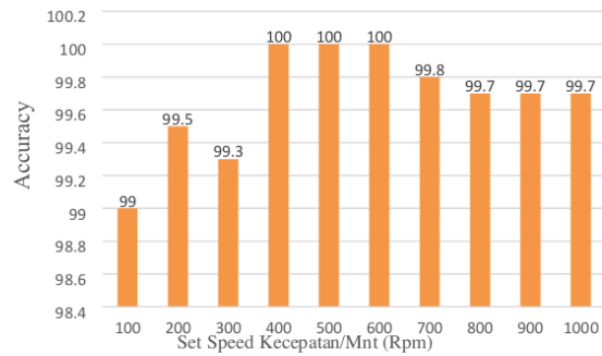
Gambar 6. Grafik Aktual Akurasi Rpm Motor
