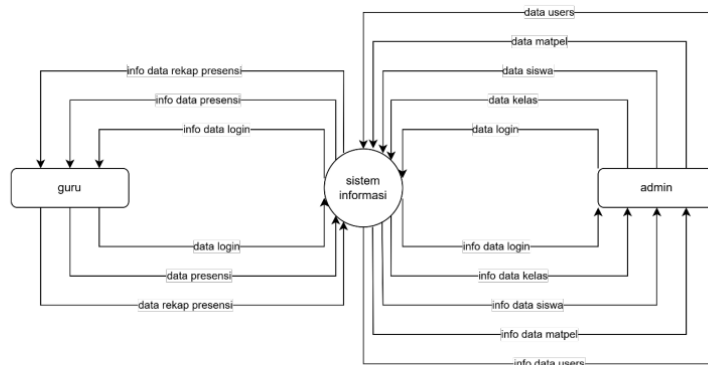
Gambar 3. DFD
