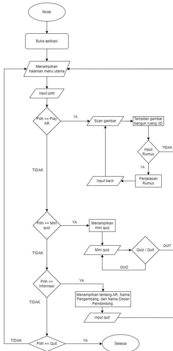
Gambar 4. Flowchart Aplikasi AR
