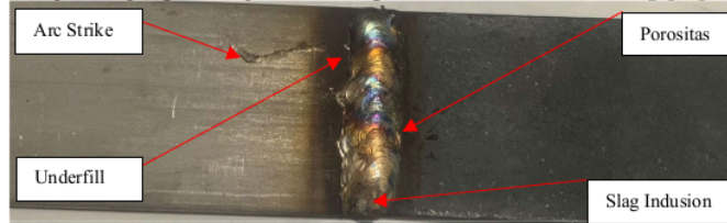
Gambar 10. Bentuk Spesimen Uji Makrostruktur
