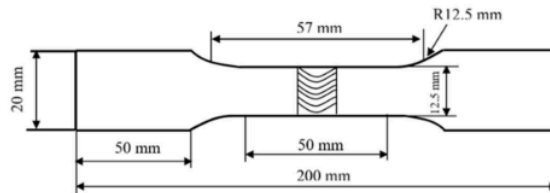
Gambar 9. Bentuk Spesimen Uji Tarik
