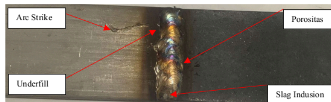
Gambar 12. Makrostruktur Spesimen 1
