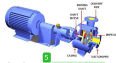
Gambar 1 Pompa Sentrifugal
