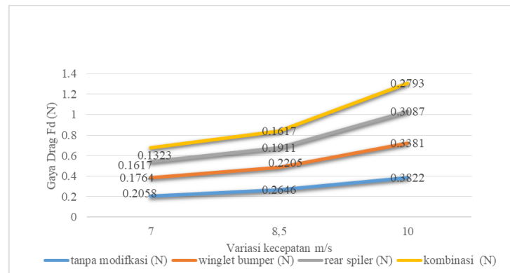
Gambar 4. Grafik nilai Gaya Drag
