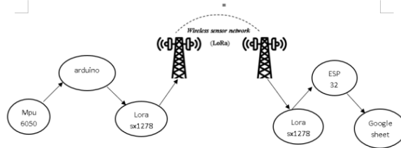
Gambar 1. Diagram blok perancangan sistem
