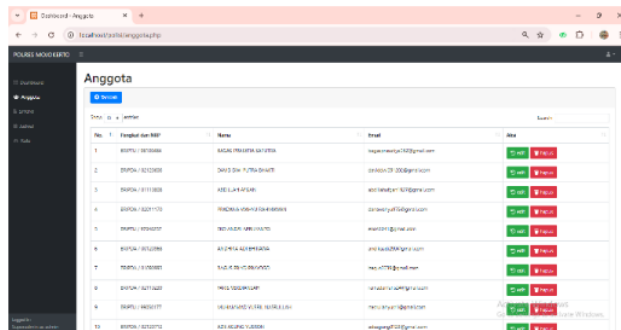
Gambar 6. Halaman Anggota
