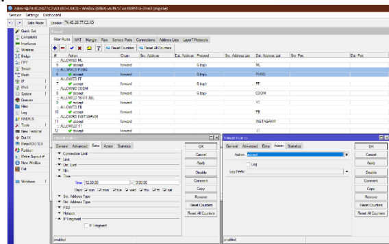
Gambar 21. Konfigurasi Extra Time Pada Firewall
