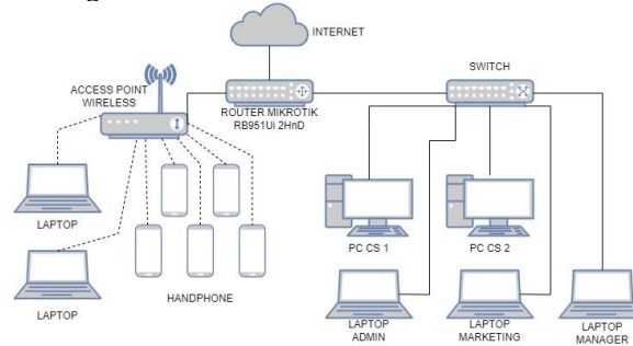
Gambar 4. Skema Topologi Baru
