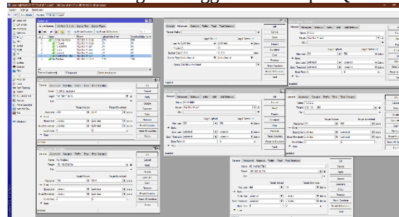
Gambar 10. Konfigurasi Limiter Bandwidth Menggunakan Simple Queue
