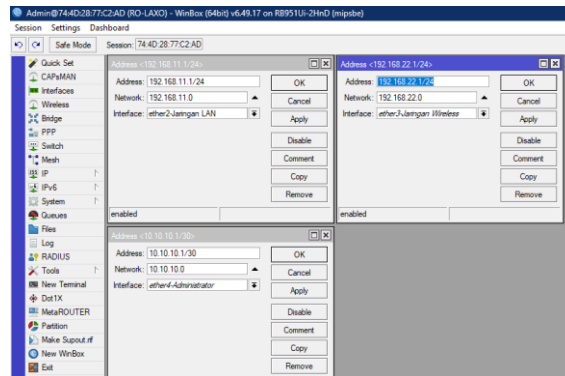
Gambar 7. Konfigurasi IP Static
