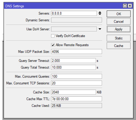
Gambar 9. Konfigurasi DNS Router Mikrotik
