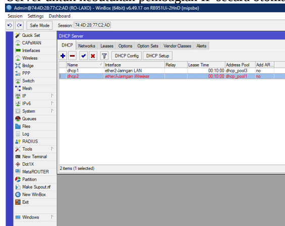
Gambar 11. Konfigurasi DHCP Server
