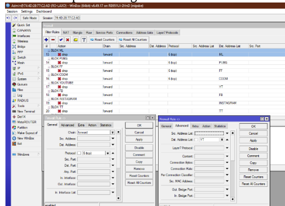
Gambar 20. Konfigurasi Blokir Pada Filter Rules Firewall
