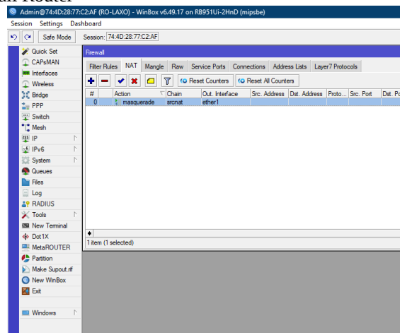
Gambar 9. Konfigurasi Firewall Pada Router
