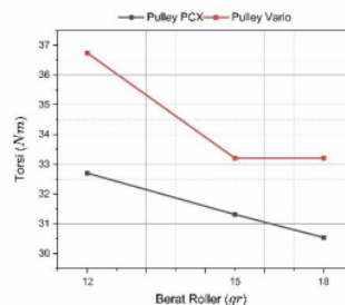
Gambar 3. Grafik Perbandingan Torsi
