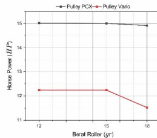
Gambar 4. Grafik Perbandingan Horse Power
