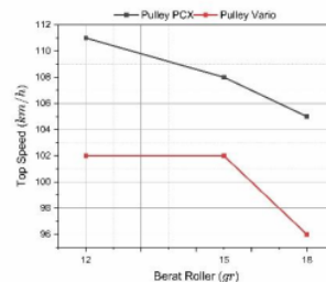
Gambar 5. Grafik Perbandingan Top Speed
