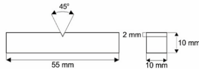
Gambar 7. Dimensi Spesimen Uji Impak
