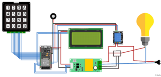
Gambar 4. Rangkaian Perangkat Keras
