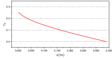
Gambar 7. Grafik Koefisien Tekanan Pada Penampang Pipa
