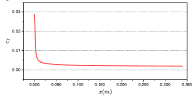
Gambar 8. Koefisien Gesek Sepanjang Permukaan Dinding Pipa
