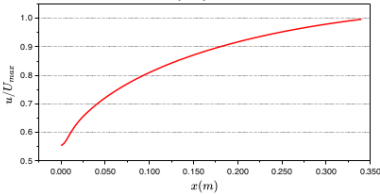
Gambar 4. Grafik Kecepatan Pada Penampang Pipa
