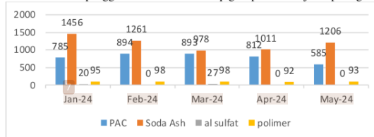
Gambar 3. GWP berdasarkan penggunaan bahan kimia
