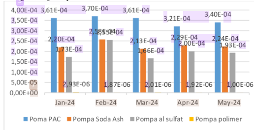
Gambar 2. GWP berdasarkan penggunaan listrik tiap bulan
