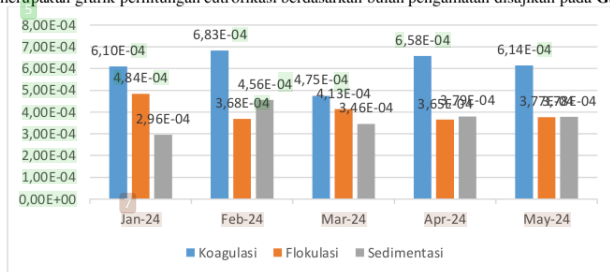
Gambar 3. Eutrofikasi berdasarkan COD
